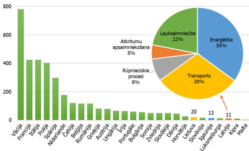
Kopējās SEG emisijas, ieskaitot netiešās CO 2 , ES valstīs (milj. tonnas) 2021. gadā un Latvijas SEG emisiju sadalījums pa nozarēm (%) 2020. gadā 3
