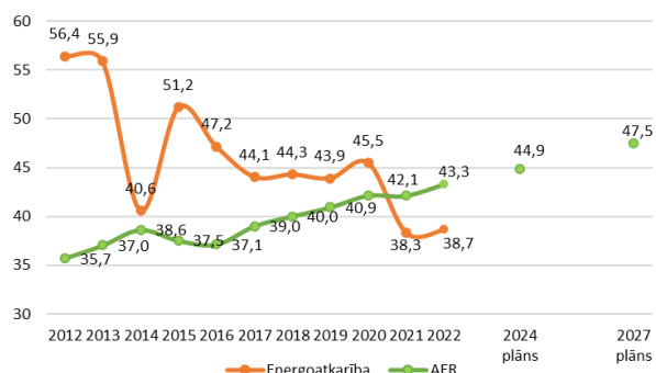
Energoatkarīga (%), atjaunīgo energoresursu (AER) īpatsvars (%) 2022. gadā un plānotās vērtības 4
