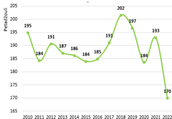
Kopējais energoresursu patēriņš 6
